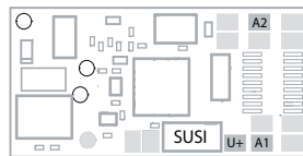
Sonderfunktionsausgänge U+, A1, A2
